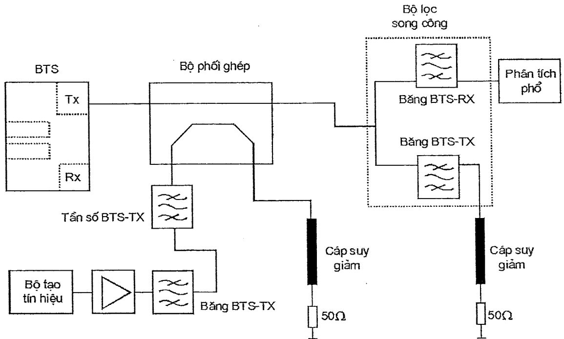
Hình A.1 - Cấu hình đo suy hao xuyên điều chế trong băng tần thu
