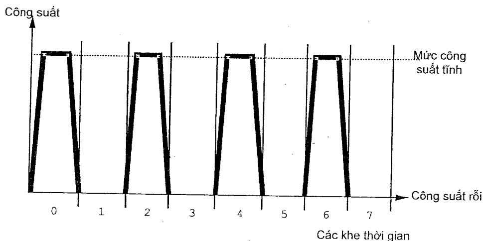
Hình 1 - Dạng công suất /khe thời gian
