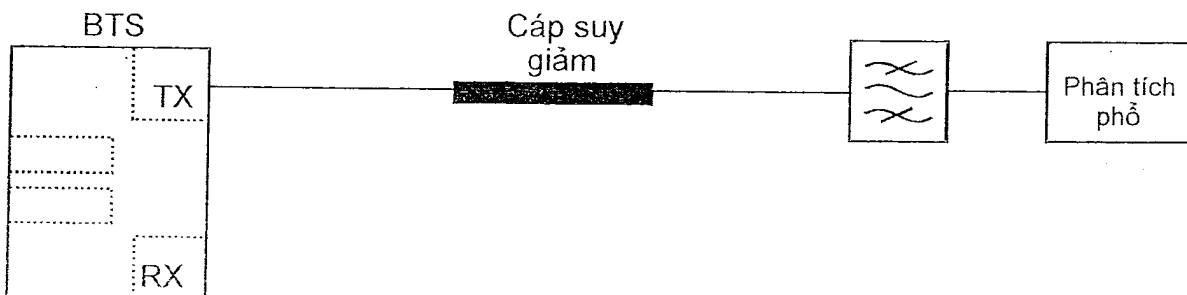
Hình A.4 - Cấu hình đo suy hao xuyên điều chế bên trong thiết bị trạm gốc trong băng tần phát
